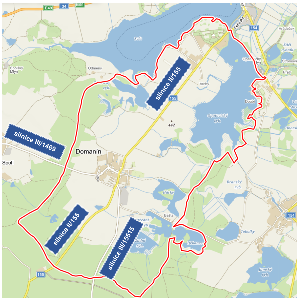
Páteřní komunikační síť v obci Domanín – krajské silnice II. a III. třídy
